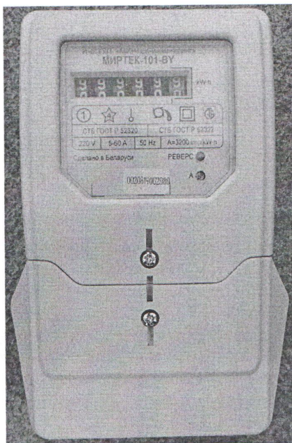
Рисунок 2 – Общий вид счетчика в корпусе модификации W1
