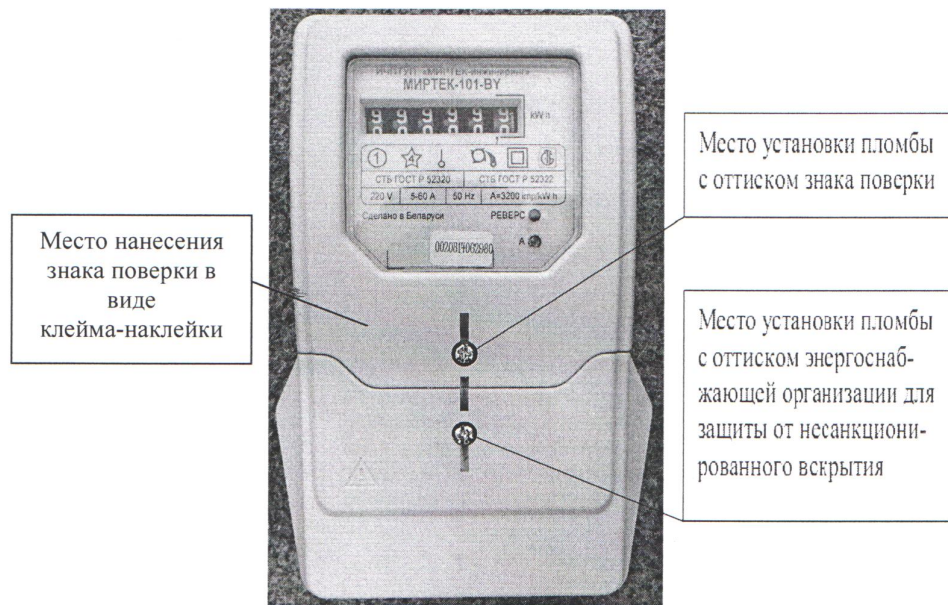
Рисунок А.1 – Места установки пломб и нанесения знака поверки для счетчиков в корпусе модификации W1
