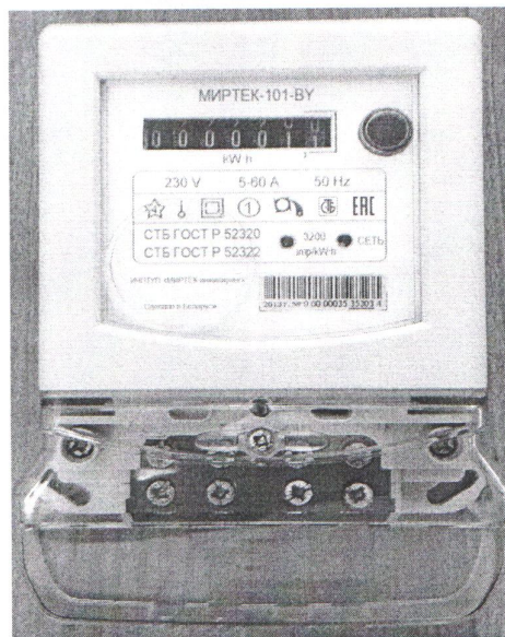
Рисунок 3 – Общий вид счетчика в корпусе модификации W2
