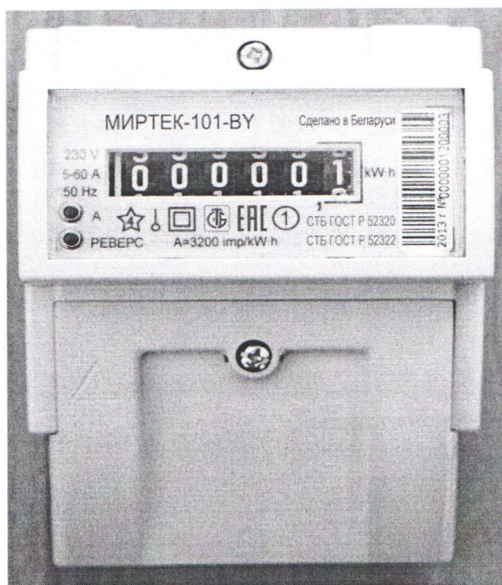
Рисунок 7 – Общий вид счетчика в корпусе модификации D5
