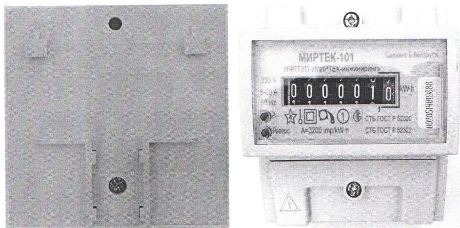
Рисунок 5 – Общий вид счетчика в корпусе модификации D3
