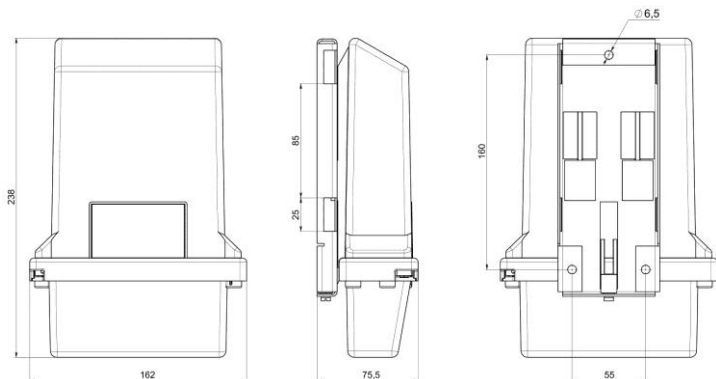
Рисунок В.1 – Внешний вид
