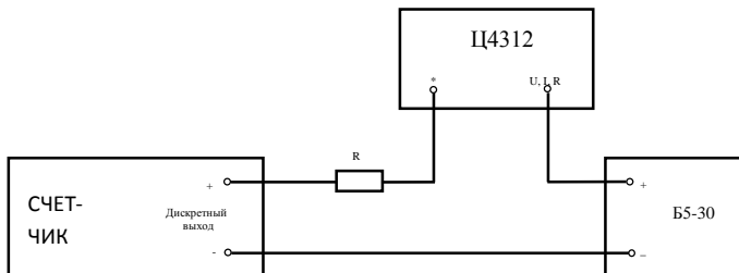
Рисунок 3.1 – Схема соединений для обеспечения функционирования испытательного устройства
