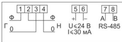
Рисунок Б.5 – Схема включения счетчиков исполнения «RS485-Q1»
