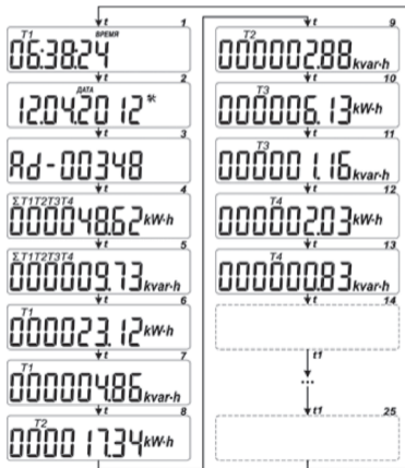
Рисунок 3.2 – Режимы циклической индикации счетчика
