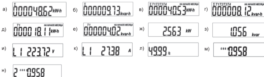
Рисунок 3.3 – Программируемые режимы индикации счетчика
