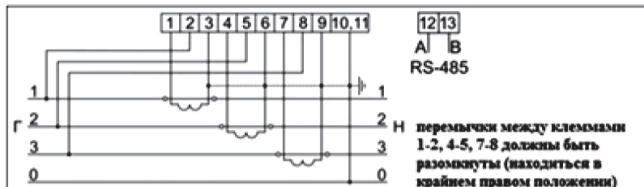
Рисунок Б.7 – Схема включения счетчиков трансформаторного включения со встроенным модулем интерфейса RS485 без дискретных выходов
