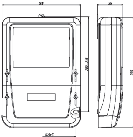
Рисунок В.1 – Счетчики в корпусе W31 для установки на щиток
